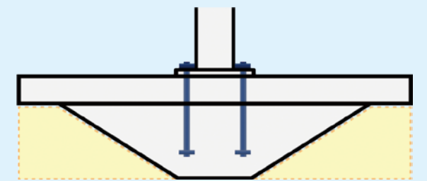
DD基礎 (4.4×4.4m)
